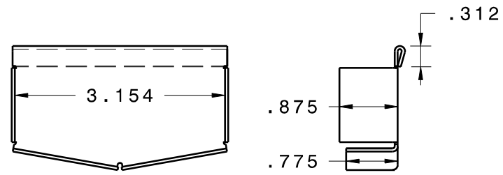
END CAP
